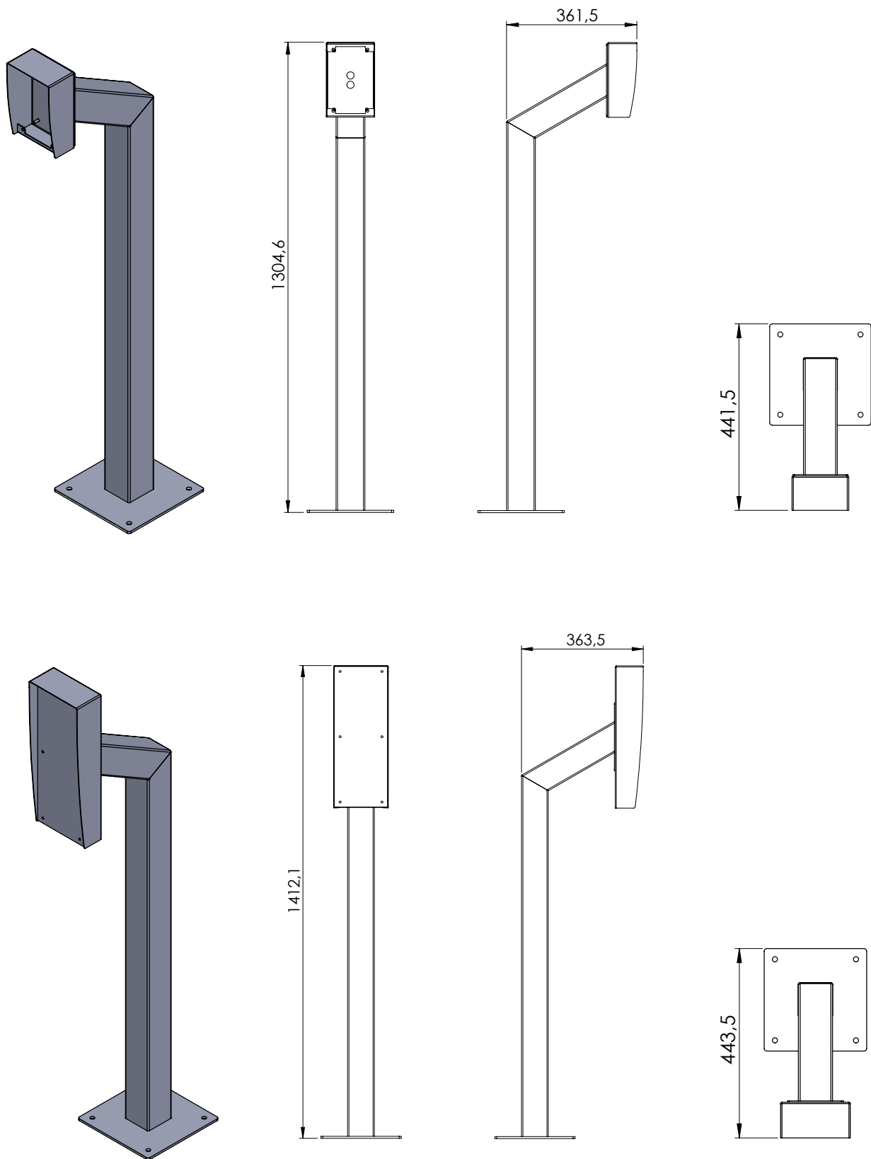
Born120Dep avec option boîtier BS420P
