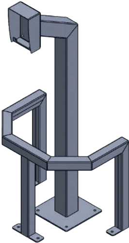
Arceau de Protection pour borne APB001
