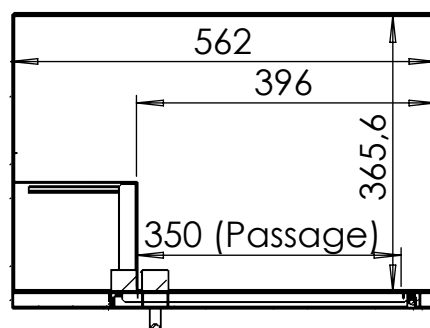
COUPE A-A
