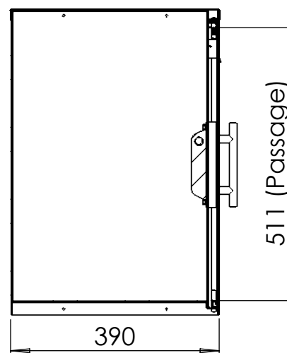
COUPE H-H
