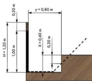
Figure B.10.1 Rampe à l'intérieur sans aménagements n'impliquant pas de hausse de l'élément de protection
