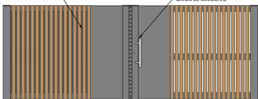
MODÈLE: GR 05 AVEC TOILE DECORATIVE ET LAMES 50x20
