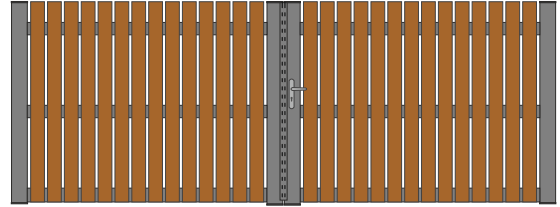
MODÈLE: GR 02 LAMES DE 100x20 EN APPLIQUE ECART +/- 20mm
