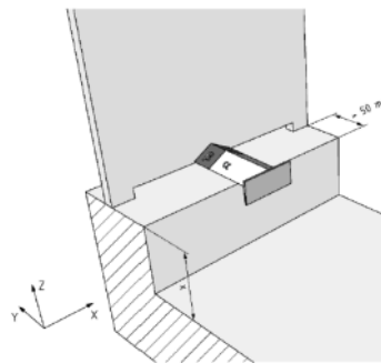
Figure B.4.1 Élément de protection comportant un appui côté intérieur La zone \alpha du gabarit B prend appui. La hauteur minimale H de l'élément de protection dépend de la hauteur x de l'appui selon le Tableau 1.
