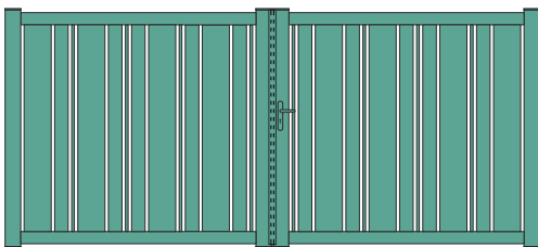
MODÈLE: AV20-100-200 LAMES ALTERNÉES VERTICALES DE 20x20 / 100x20 / 200x20
