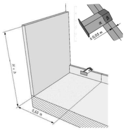
Figure B.4.2 Élément de protection avec muret ne constituant pas un appui Seule la zone \beta du gabarit B prend appui. La zone \alpha ne prenant pas appui, il n'est donc pas nécessaire de rehausser l'élément de protection.
