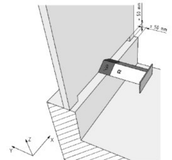
Figure B.4.2 Élément de protection avec muret côté intérieur, ne constituant pas un appui. Seule la zone \beta du gabarit B prend appui. La zone \alpha ne prenant pas appui, il n'est donc pas nécessaire de rehausser l'élément de protection
