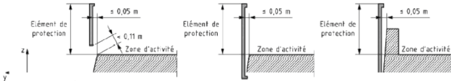
Figure 18 Dispositions complémentaires de sécurité en partie inférieure de l'élément de protection
