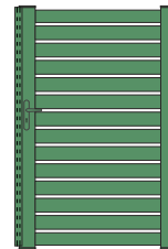
MODÈLE: CH100 LAMES HORIZONTALES DE 100x20 AJOURÉS
