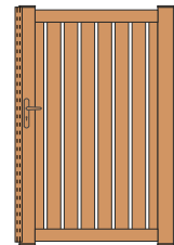
MODÈLE: CV100 LAMES VERTICALES DE 100x20 AJOURÉS
