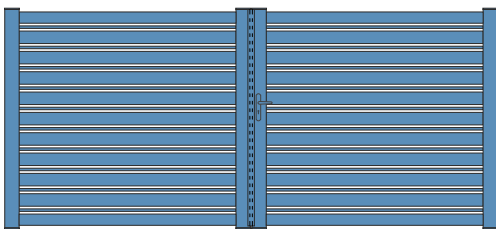
MODÈLE: CH20-100 LAMES ALTERNÉES HORIZONTALES DE 20x20 / 100x20
