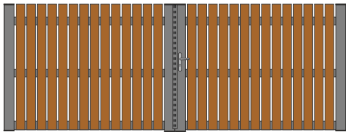
MODÈLE: GR 02 LAMES DE 100x20 ECART +/- 20mm
