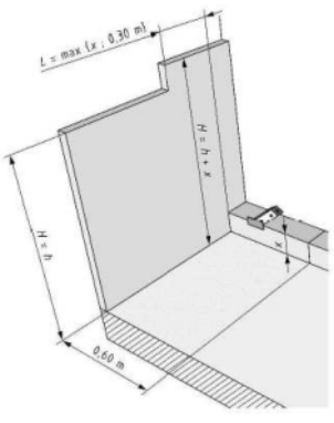
Figure B.4.1 Élément de protection avec muret constituant un appui La zone \alpha du gabarit B prend appui. La hauteur minimale H de l'élément de protection dépend de la hauteur x de l'appui selon le Tableau 1.
