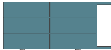
COULISSANT AVEC 6 TÔLES HORIZONTALES + REMPLISSAGE DE LARGEUR MAXI 5000mm
