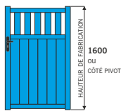
Forme A LAMES 150 VERTICALES
