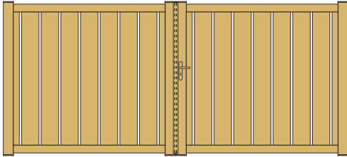
MODÈLE: CV200 LAMES LARGES VERTICALES DE 200x20 AJOURÉS
