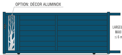
MODÈLE V04 ASPECT 2 VANTAUX SIMPLIFIÉS AVEC 1 MENEAU CENTRAL
