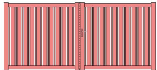
MODÈLE: AV20-100 LAMES ALTERNÉES VERTICALES DE 20x20 / 100x20
