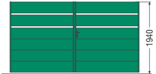
Y3 - Lames de 300 avec 2 ajour de 50mm entre 2 lames.
