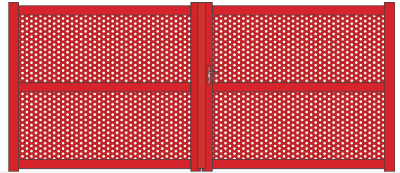
DIVES D2 - TÔLE PERFORÉE RONDE RÉF. R5T8
