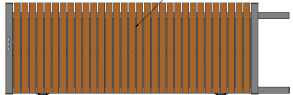
MODÈLE: GR 02 LAMES DE 100x20 ECART +/- 20mm
