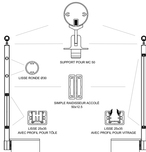
GARDE CORPS AVEC VITRAGE, MAIN COURANTE RONDE POSE EN APPLIQUE
