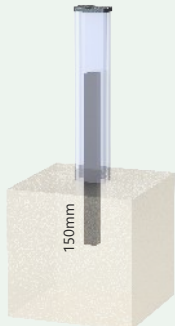
POTEAU 76x41 à sceller avec tube 30x30 acier Longueur 500mm Hauteur maxi conseillée 1.100mm
