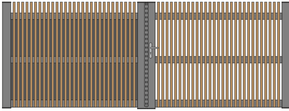
MODÈLE: GR 01 BARREAUX 30x30 OU 50x20 EN APPLIQUE ECART +/- 20mm
