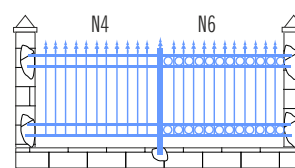
N4 N6 4 TRAVERSES 40x20 ou MÉPLAT 40x10 2 RANGÉES DE RONDS
