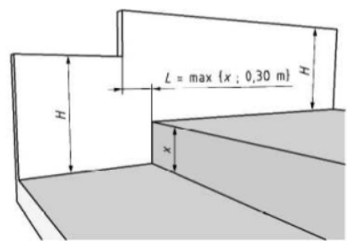
Figure 13- Prolongement lateral dû à un dénivelé
