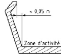
Figure 19 Dispositions complémentaires de sécurité de l'élément de protection galbé ou incliné vers l'extérieur
