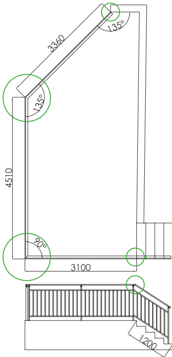
Plan du génie civil mesures hors tout (voir notre relevé de côte)
