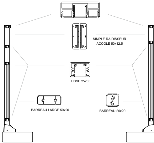
GARDE CORPS BARREAUDÉ LARGE, MAIN COURANTE RECTANGULAIRE POSE SUR DALLE
