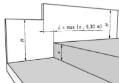
Figure 13 Prolongement latéral dû à un dénivelé
