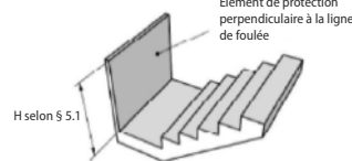
Figure 16 Eléments de protection non rampants et perpendiculaires à la ligne de foulée des escaliers
