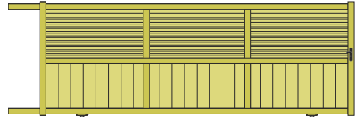
3 DIVISIONS AVEC 2 MENEUX VERTICAUX
