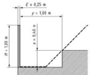
Figure B.10.2 Rampe à l'intérieur avec aménagements nécessitant la hausse de l'élément de protection
