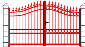
• DOUBLE TRAVERSE INTERMÉDIAIRE • 2 RANGÉES DE ROUNDS • DOUBLE TRAVERSE HAUTE CDG
