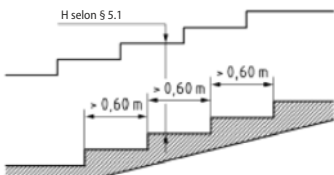
Figure 15 Succession de paliers de profondeur > à 0,60 m
