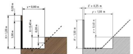
Figure B.10.2 Exemple d'un dénivelé dans la zone d'activité impliquant une rehausse de l'élément de protection
