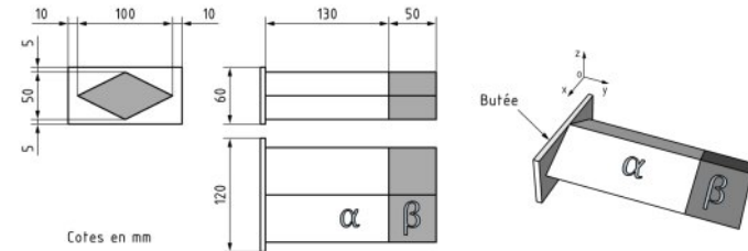
Figure 6 Gabarit B permettant la détermination des appuis (vis-à-vis du risque de basculement)
