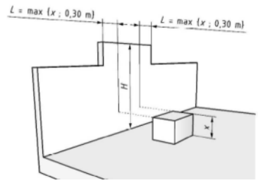
Figure 12 - Prolongement latéral dû à un appui entrainant une rehausse de la hauteur minimale de protection
