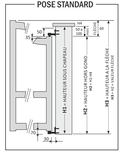
HAUTEUR AU GOND +/- 60 mm
