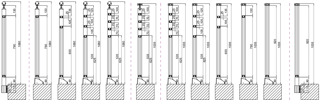
SEPARATIFS À LISSES
