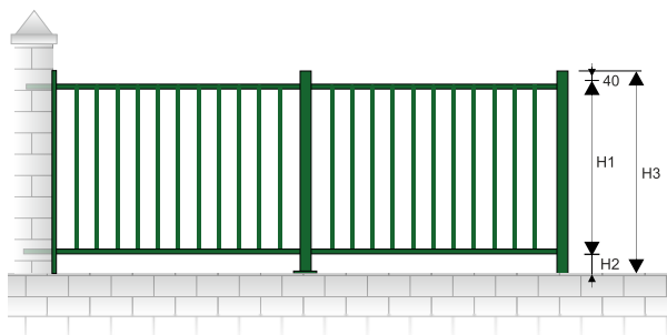
Clôture Barreaudée City 2 traverses sans fer de lance
