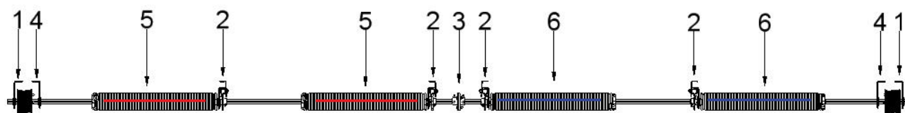
Arbre avec quatre ressorts de torsion.
