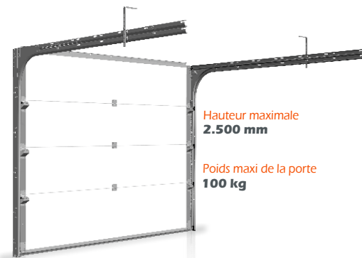
RES70 Ressort à Extension (RESSORT LATÉRAL)
