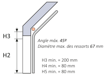
INCLINÉ RES200i
