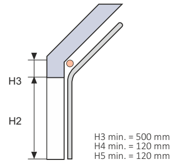
INCLINÉ IND-IL
