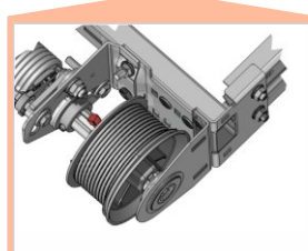
RES100 Linteau Réduit (RESSORT ARRIÈRE)
