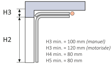
RÉDUIT RES100
