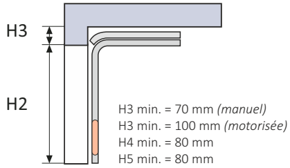
RESSORT À EXTENSION RES70x / RES100xm
