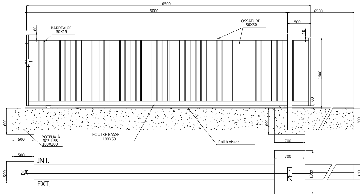
PORTAIL A25 COULISSANT (GAMME UTIL) DROIT 6000 AVEC SERRURE
