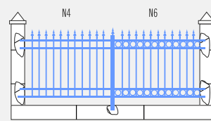
4 TRAVERSES 40x20 OU MEPLAT 40x10
